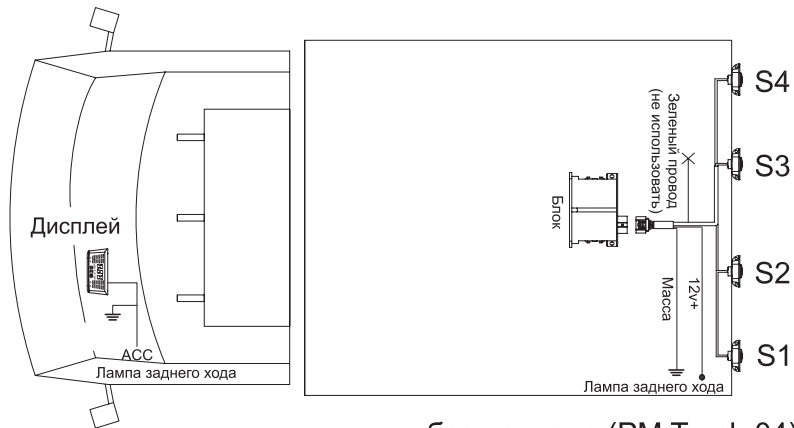
без прицепа (PM Truck-04)
